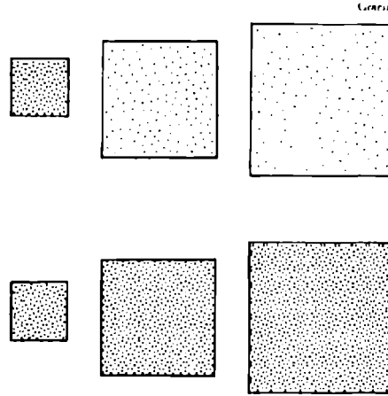
3 - يناقش هذا الشكل ثلاث لقطات متتالية لمنطقة في الفضاء المتوسع إبان الانفجار الكبير، ونماذج لحالات ثابتة للكون "في حالة الانفجار الكبير (الأعلى)، يبقى عدد
