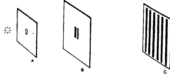
14 - إن تجربة يونغ الشهيرة "نظام الشقين"، نموذج لعرض الثنائية العجيبة للضوء؛ الموجة - الجسم (يمكن أيضاً تنفيذها مع الإلكترونات، أو جسيمات أخرى).
