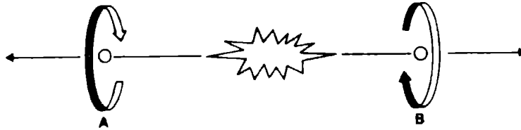
11 - إن اضمحلال ذرّة ما، أو جسيم ذري، يمكنه إنتاج جزعين اثنين، يدوران بشكل معاكس، بما يشابه فوتونات الضوء التي تسافر في اتجاهين معاكسين، وربّما إلى مسافة كبيرة.
